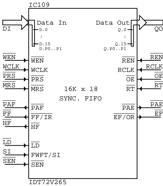
IDT72V265
