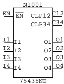
75438NE N????
